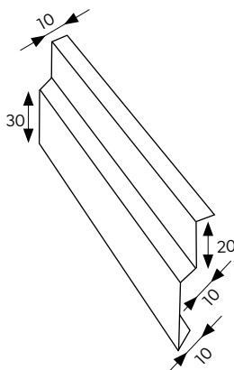
DILATÁCIÓS LÉC
